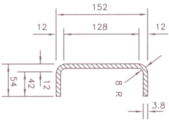
SECTION D-D
