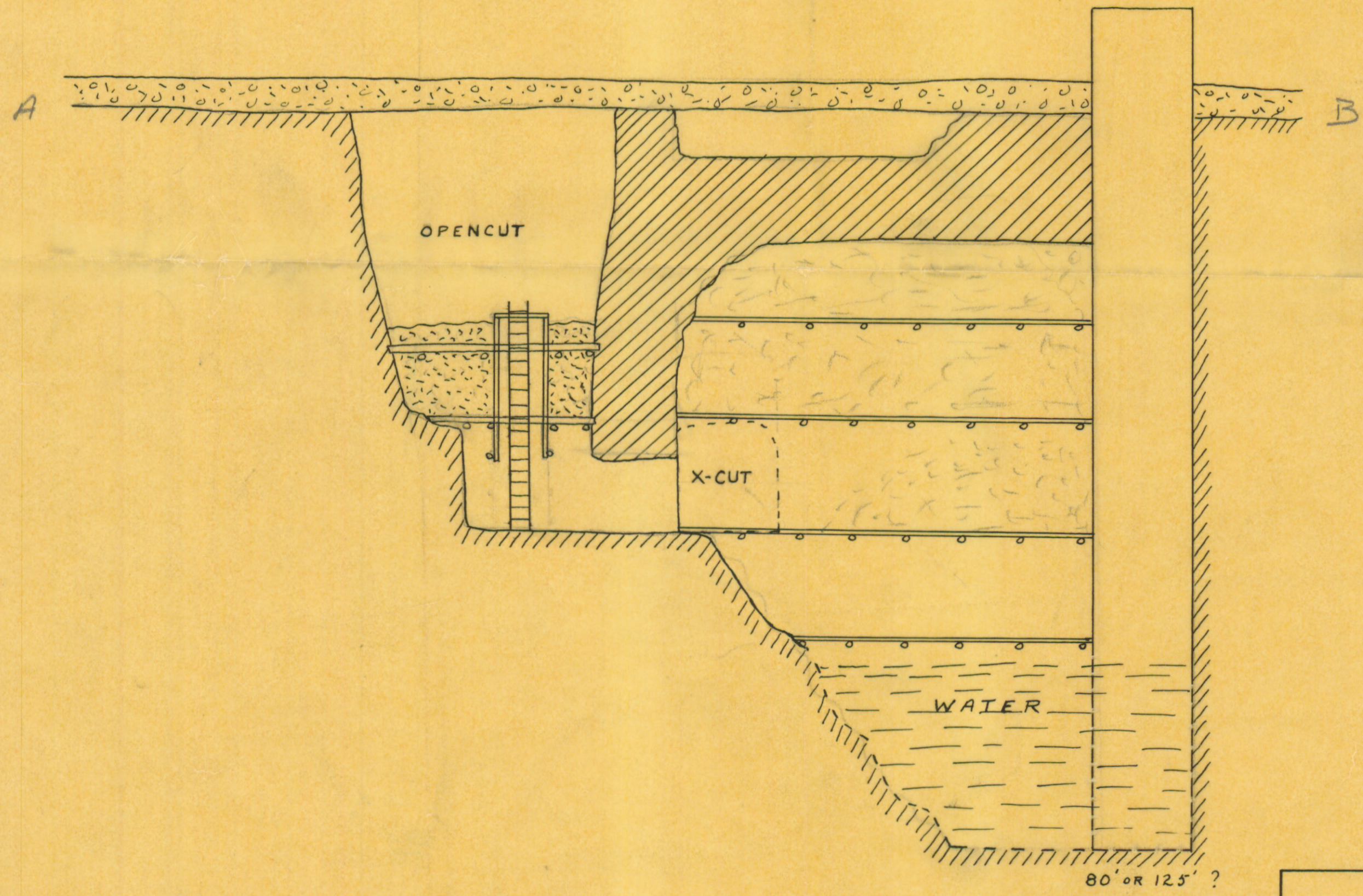
LONGITUDINAL SECTION
