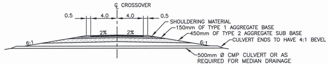
SECTION A-A
