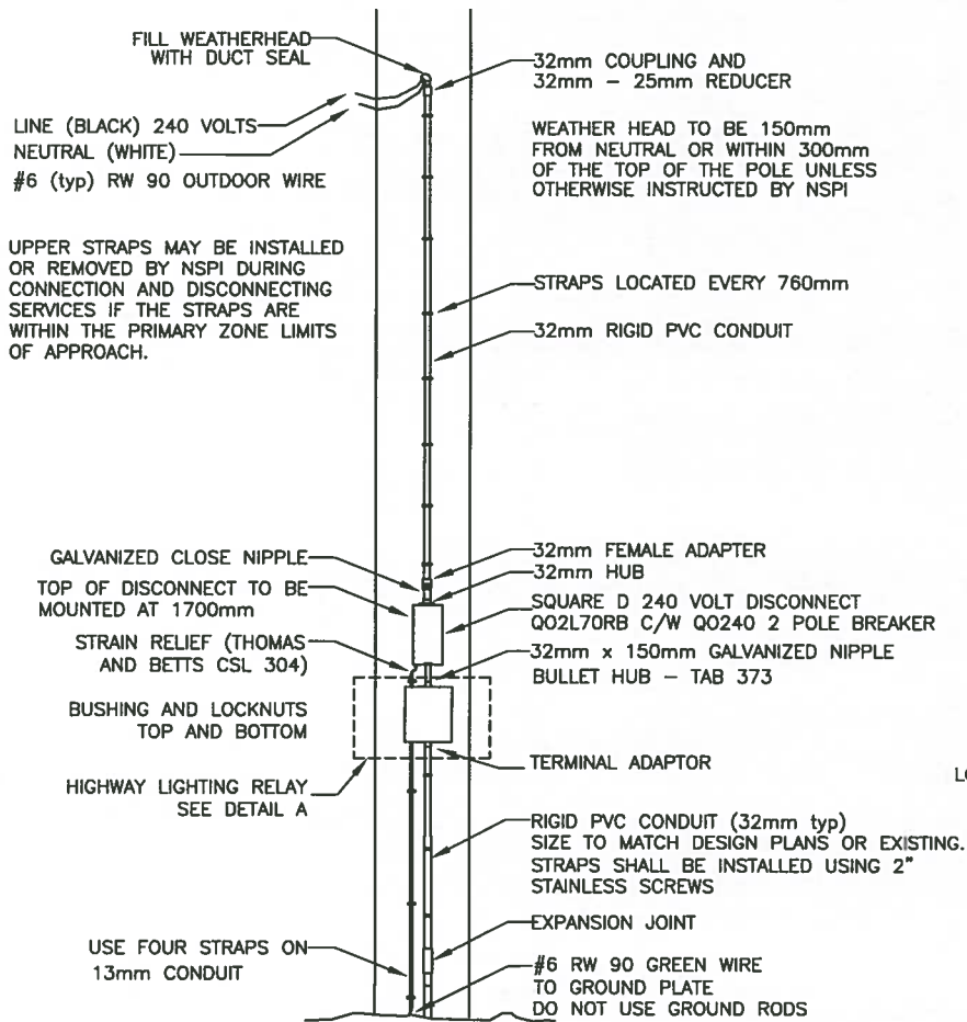
TYPE B SERVICE - 240 VOLT C/W RELAY
